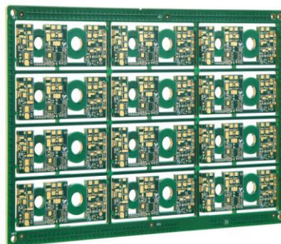
高多层厚铜板+工控
