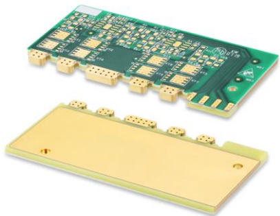
嵌铜块+侧壁金属化 大功率电源板-通信
