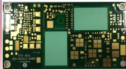
单层双面铝基板+激光盲孔+电源板
