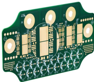
嵌铜块+汽车照明
