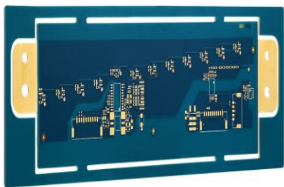
含导热绝缘树脂的双面夹芯板+汽车照明/电源
