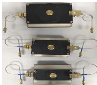
矢量网络分析仪 + Dk、Df测试系统
